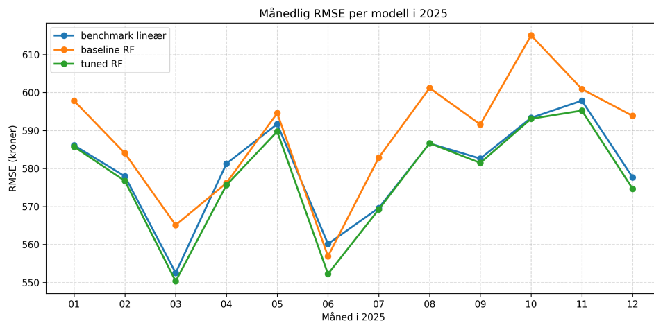
Figur 9: Figur 7.2 Månedlig RMSE per modell i 2025. Tuned Random Forest har lavest RMSE i majoriteten av månedene, mens benchmark lineær slår gjennom i enkeltmåneder.
